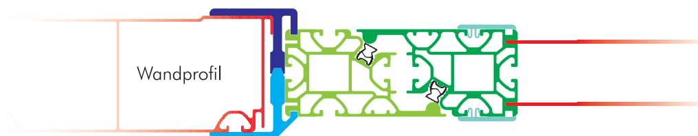
Türhaltewinkel innen
