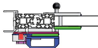
Türblendenprofil 40
